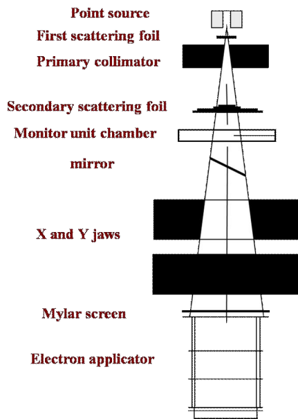
شکل ۱- مولفه های سر شتابدهنده
