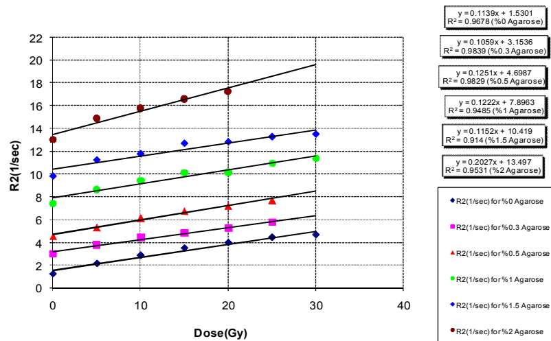
شکل ۱- نمودار تغییرات R2-dose در ژل PAGATA با درصد‌های وزنی مختلف آگارز
