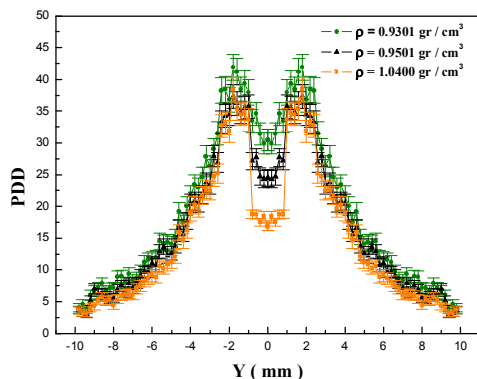
شکل ۴- تغییرات درصد دوز عمقی در راستای Z=3 میلیمتر.
