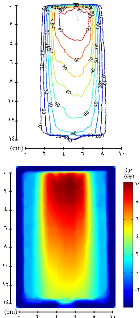
شکل ۴ - منحنی های همدوز و نقشه ی دوز در فانتوم استوانه ای که با استفاده از ژل دوزیمتری به دست آمده است (تک میدان)
