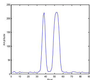
الف) پروفایل فانتوم Jaszak شبیه سازی شده
