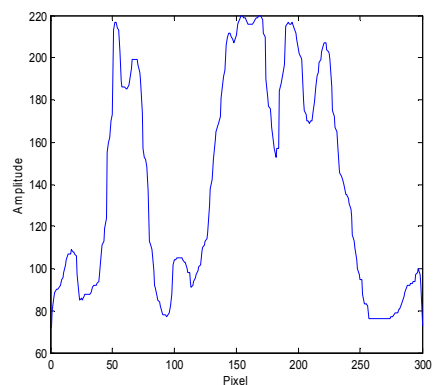
ج) پروفایل تصویر قلب نویززدایی شده پس از اعمال فیلتر میانگین (5*5)
