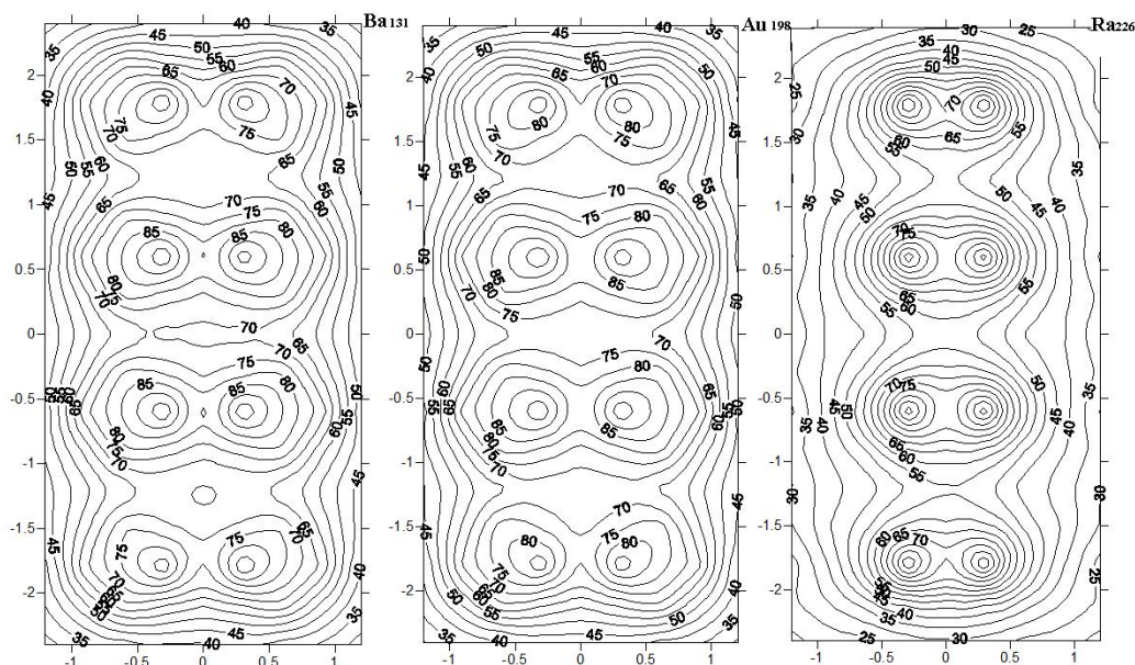
شکل ۱- مقایسه توزیع دوز در اطراف چشمه های مختلف (مقادیر ذکر شده در شکل به صورت درصدی می باشند)
