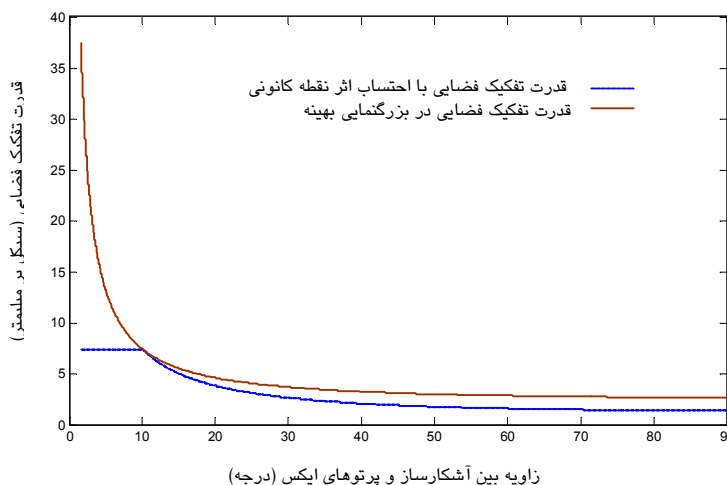
شکل ۸- مقایسه قدرت تفکیک فضایی سی تی با احتساب اثر نقطه کانونی ۶/۷۰ میلیمتر و با بهینه کردن ضریب بزرگنمایی
