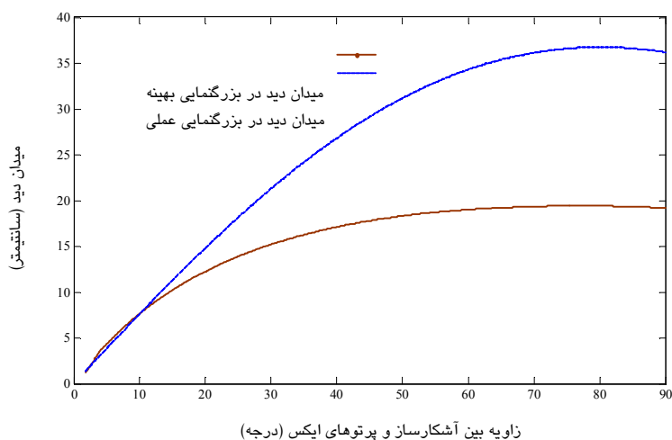
شکل ۹- مقایسه میدان دید دستگاه در بزرگنمایی بهینه و بزرگنمایی ثابت عملی
